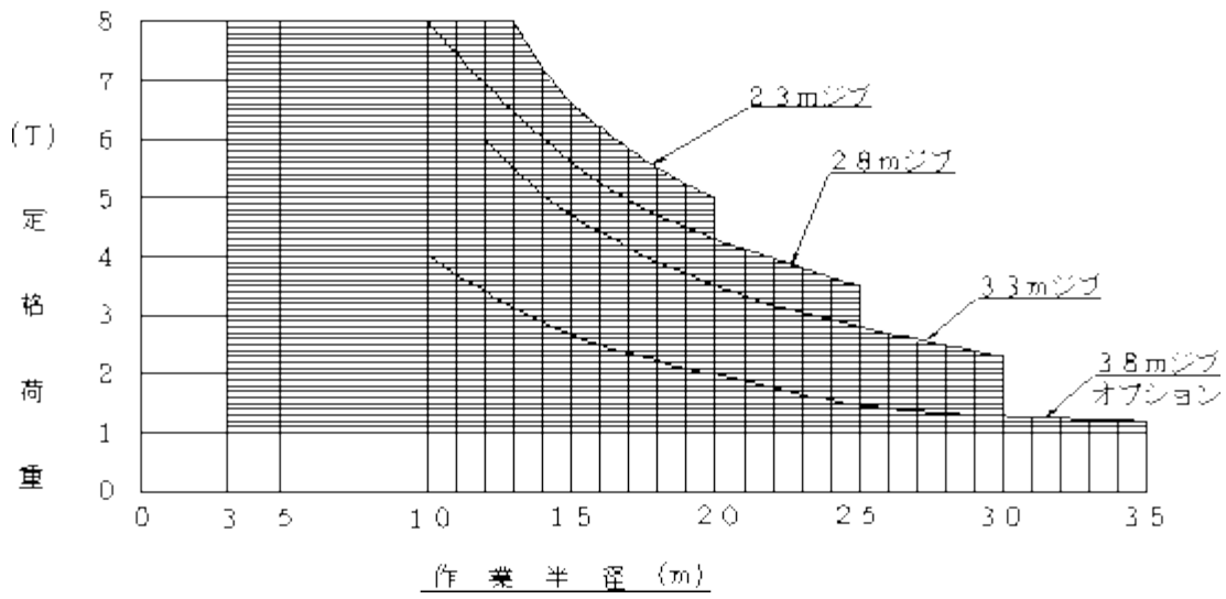
性能曲線図
